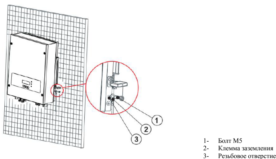
Рисунок 17 Подключение заземления
