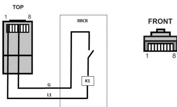
Рисунок 38 Инвертор – RRCR соединение
