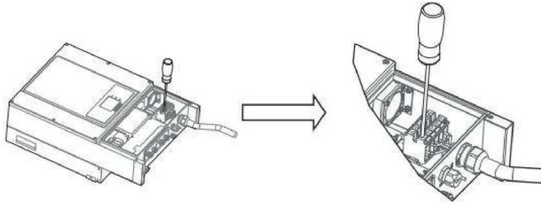
Рисунок 26 Обработка кабеля
