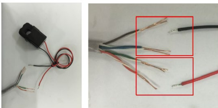
Рисунок 34 Подключение трансформатора тока кабелем UTP
