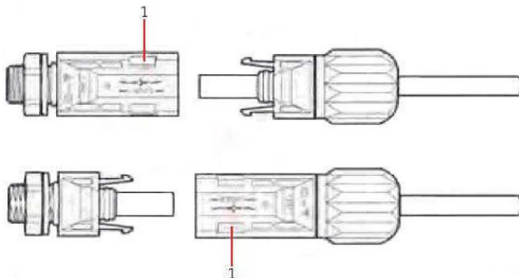
Рисунок 22 Подключение кабелей входной мощности постоянного тока (DC)
