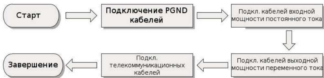
Рисунок 14 Блок-схема для подключения проводов к инвертору
